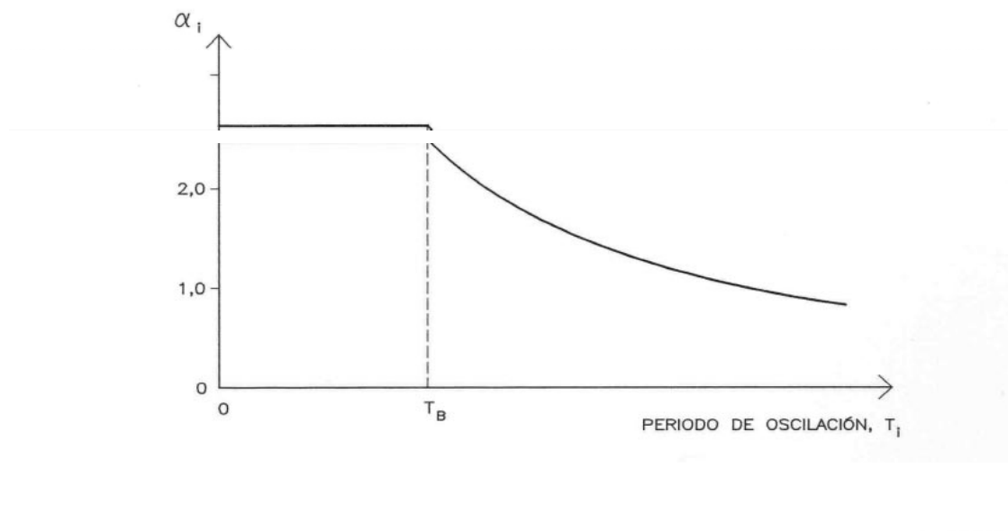
Figura 3.3. Coeficiente \alpha_i para el método simplificado de cálculo.
