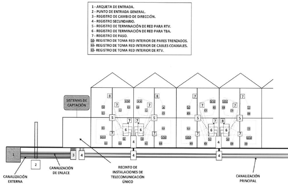
APENDICE 9: Infraestructura para viviendas unifamiliares
