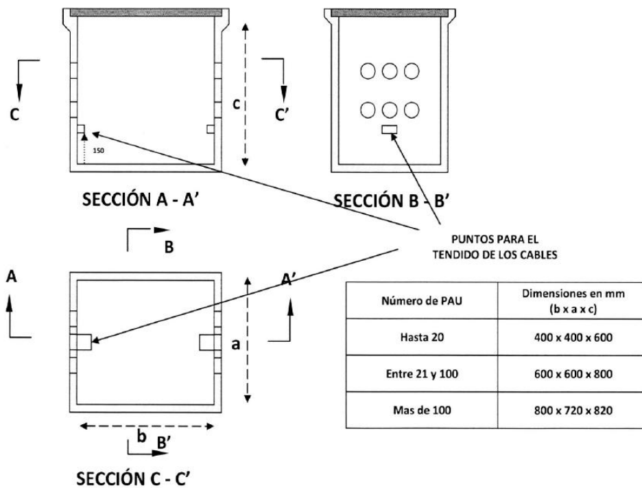
APENDICE 3: Dimensiones mínimas de la arqueta de entrada
