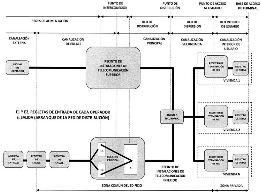
APENDICE 1: Esquema general de una ICT
