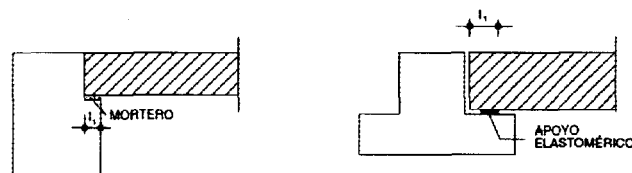
Figura 21.3.1 Apoyos directos de losas alveolares
