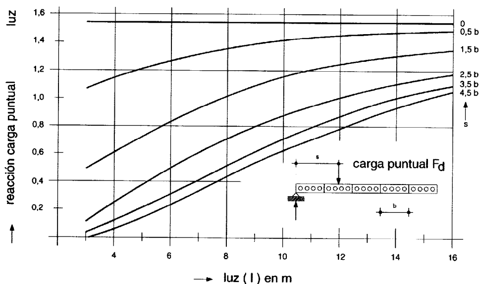
Figura A.3.6 Fuerza de reacción en el apoyo longitudinal debida a una carga puntual en el centro de vano
