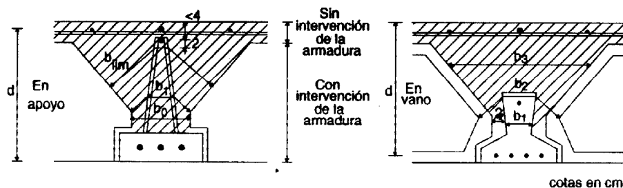
Figura 14.2.1.a Comprobación de esfuerzo cortante con piezas de entrevigado aligerantes
