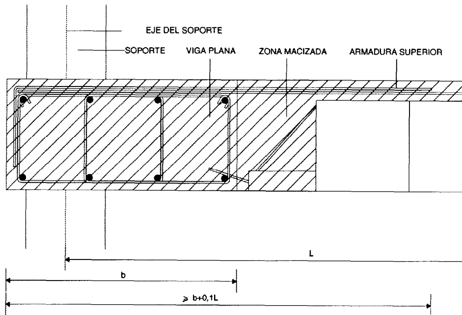
Figura 22.a Anclaje de armadura superior en extremo
