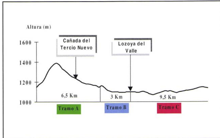
Perfil topográfico
