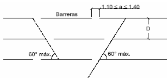
Figura 2.1 Líneas sucesivas de barreras en planta
