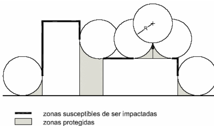
Figura B.3 Esfera rodante en estructuras
