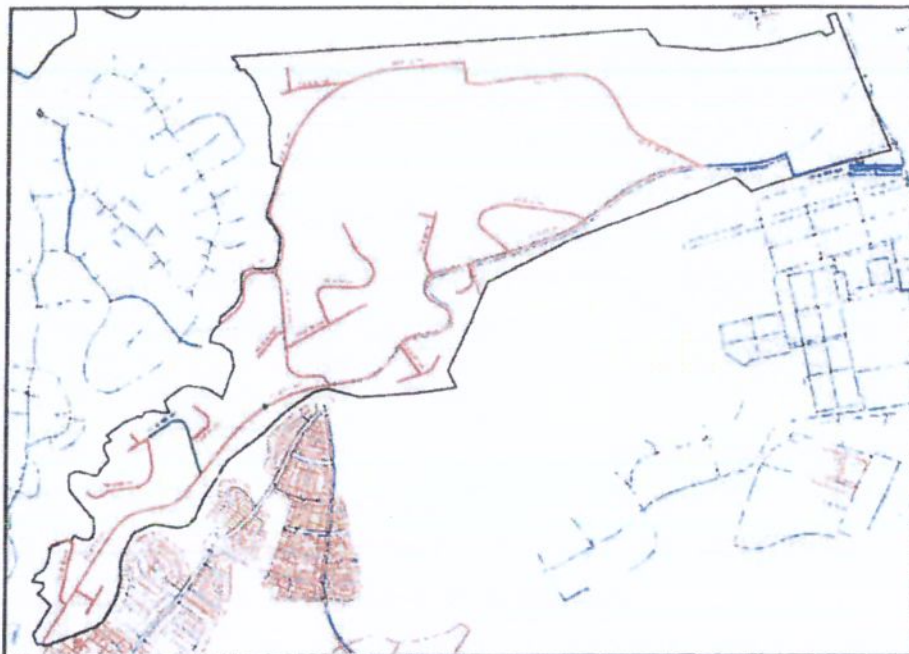
Esquema de red de distribución propuesta. Red de gravedad. — Ø 80 mm. — Ø 100 mm. — Ø 150 mm. — Ø 200 mm.
