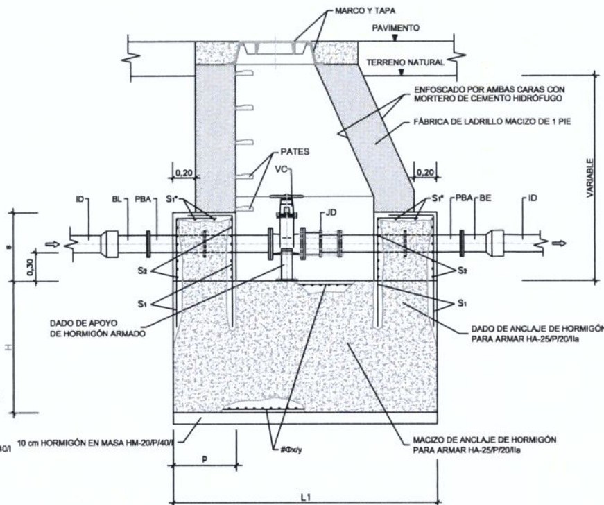
SECCIÓN LONGITUDINAL SIN ESCALA
