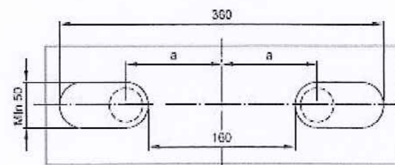
ORIFICIOS DE ENTRADA Y SALIDA DE TUBERÍAS DE ACOMETIDAS EN ARMARIOS DE CONJUNTO DE MEDIDA
