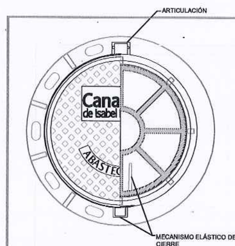
TAPA Y MARCO CON BISAGRA Y CON DISPOSITIVO DE ACERROJADO Y ANTIRROBO
