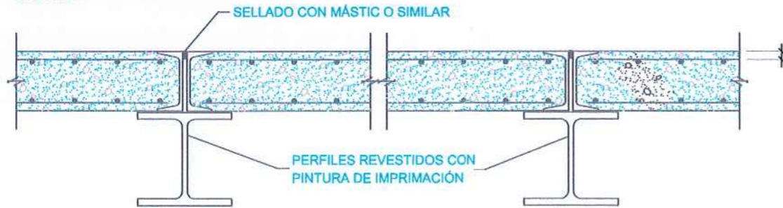
SECCIÓN B-B
