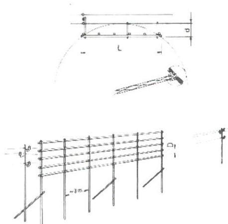
Fig. 8: D) Distancia entre traviesas igual a 0,5 m d) Distancia de pantalla a L.E. de 5m si la tensión es superior o igual a 50 Kv y de 3 m si es menor.
