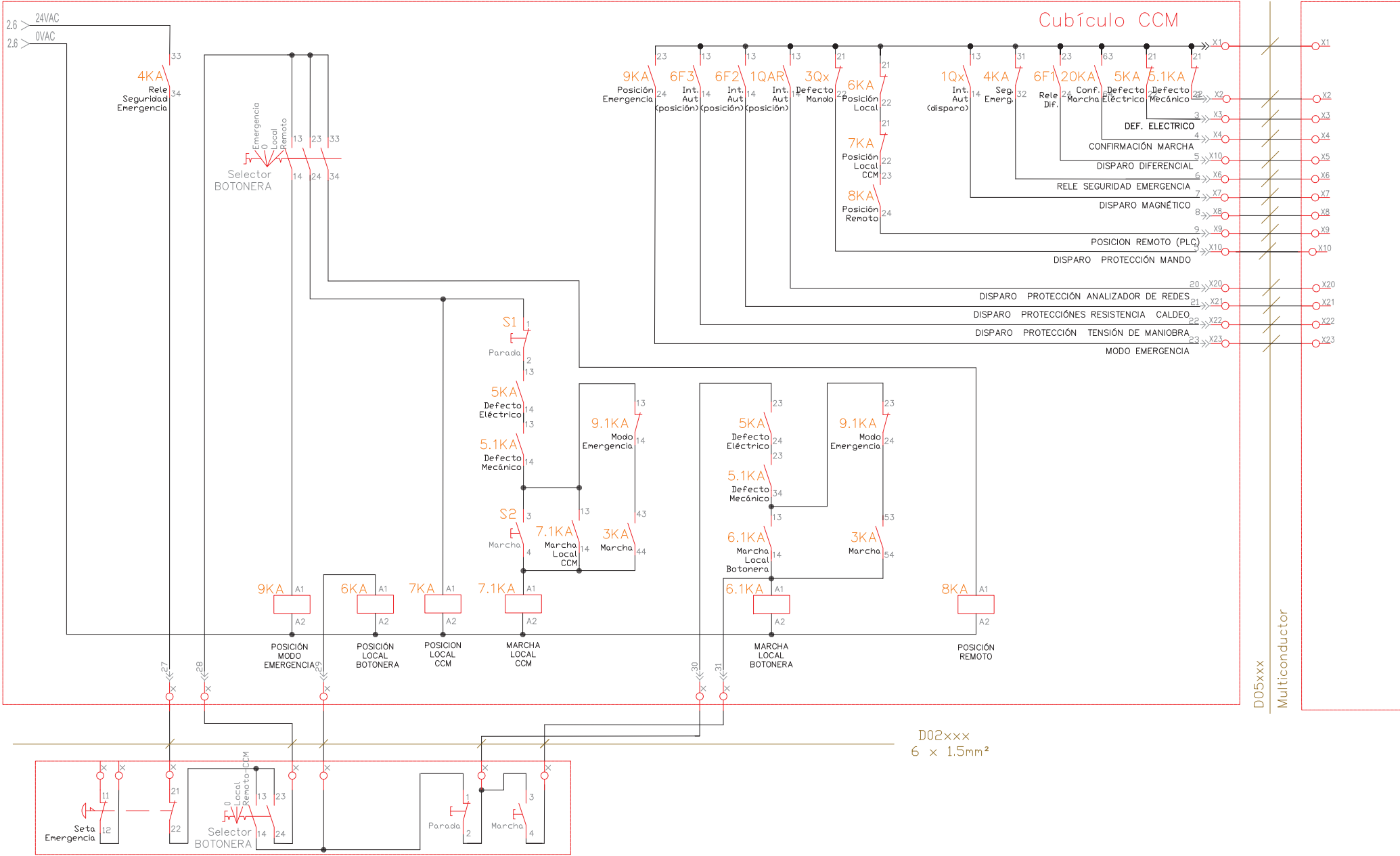
BOTONERA A PIE DE MÁQUINA
