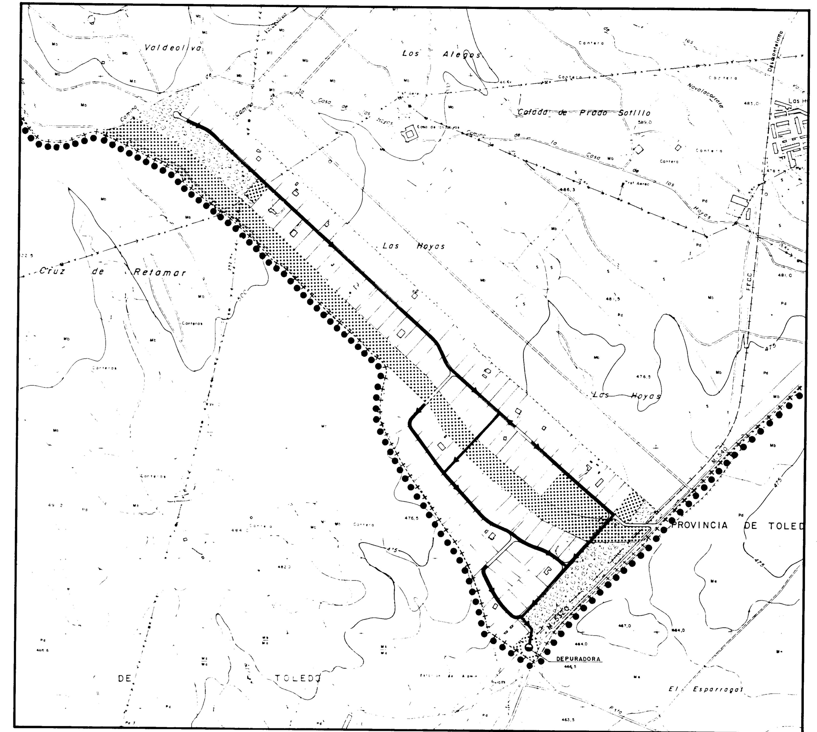
ESQUEMA DE LA RED DE SANEAMIENTO DEL P.O.N.P. "LAS HOYAS"
